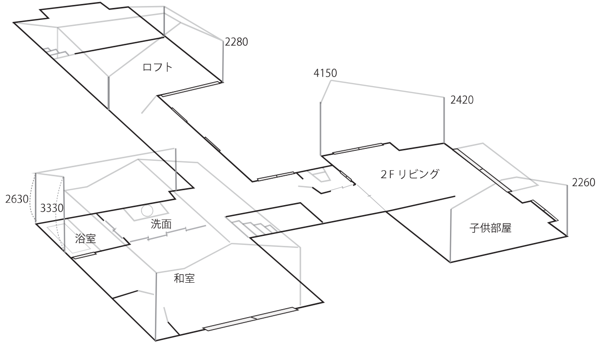
天井高図面
